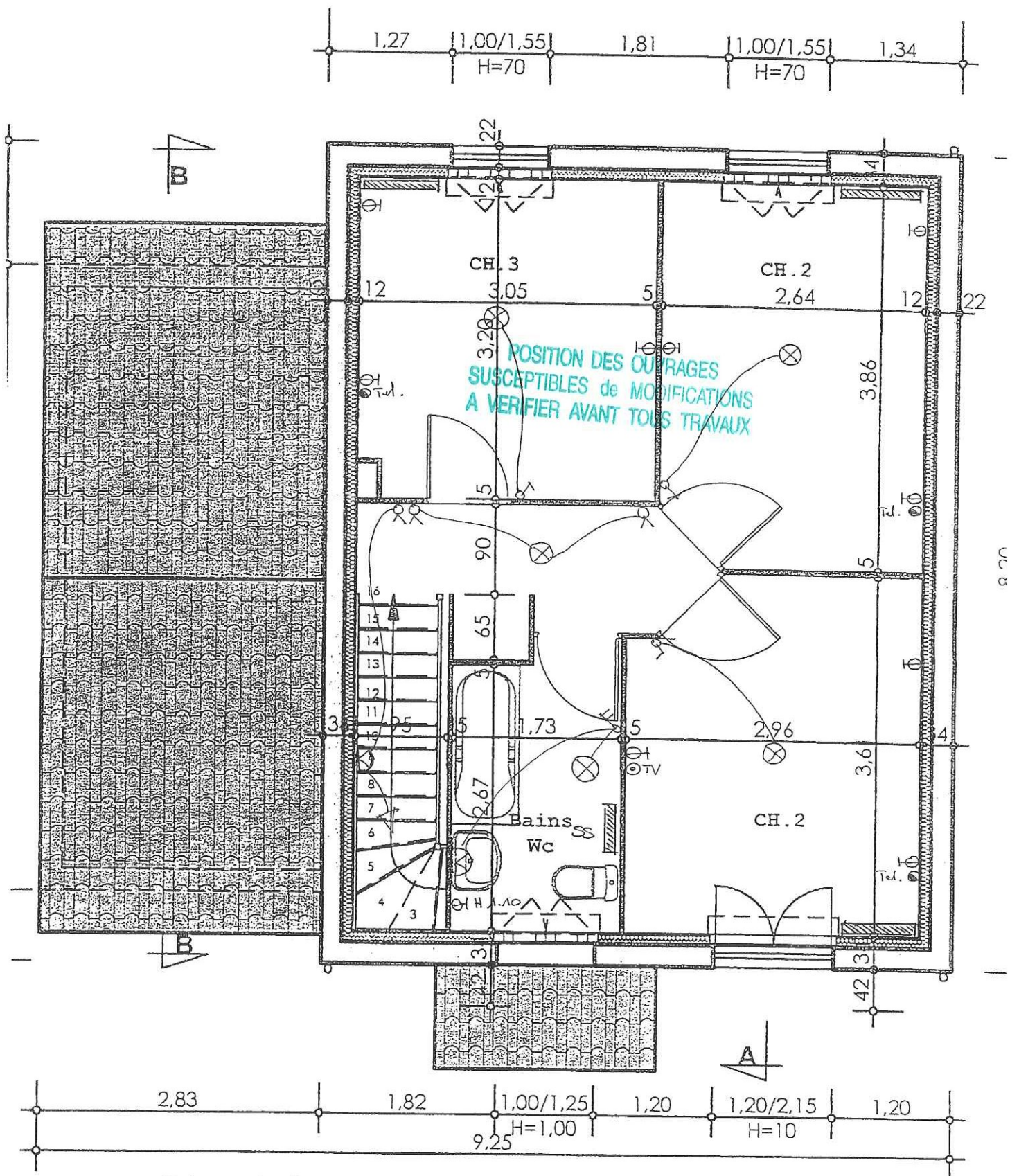
PLAN ETAGE
